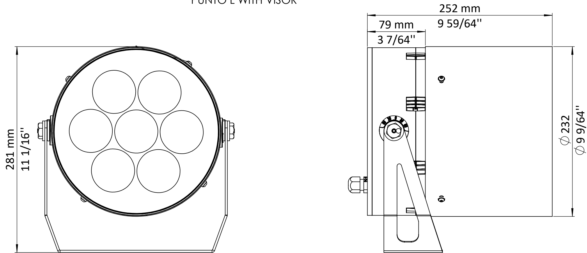
PUNTO L WITH VISOR
