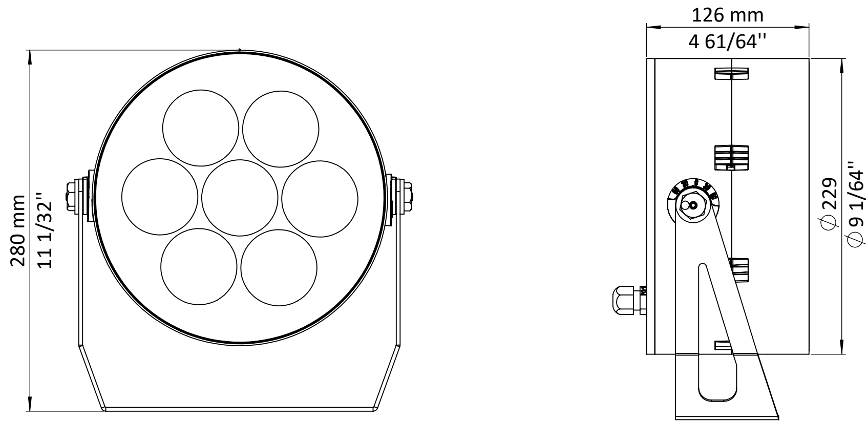
PUNTO L WITHOUT VISOR
